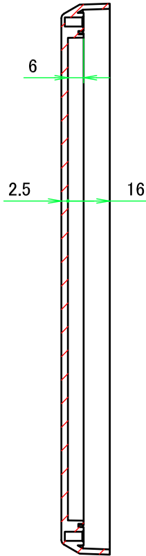
C-C ( 1 : 2 )
